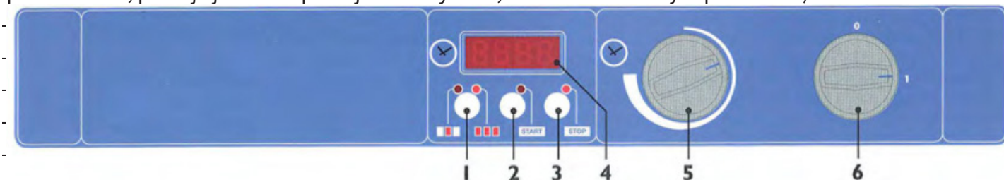
Obr. 1: Nastavení jednotky. 1 - Digitální displej, 2 - Vypínač jednotky, 3 - Start, 4 - Stop, 5 - Výběr topného článku, 6 - Nastavení teploty.
